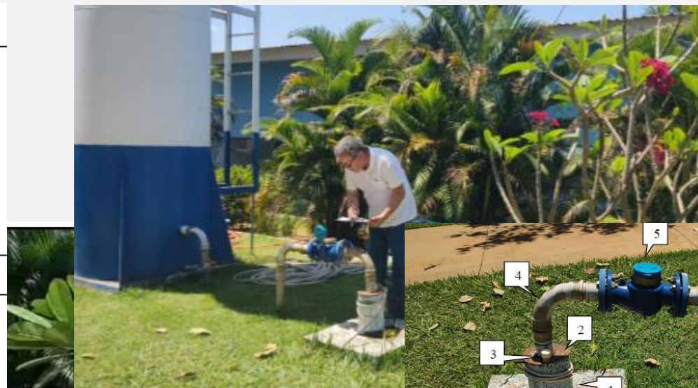
Ensaio de bombeamento para determinação da vazão – hidrômetro F25AK0001366 de 30 m³/h
